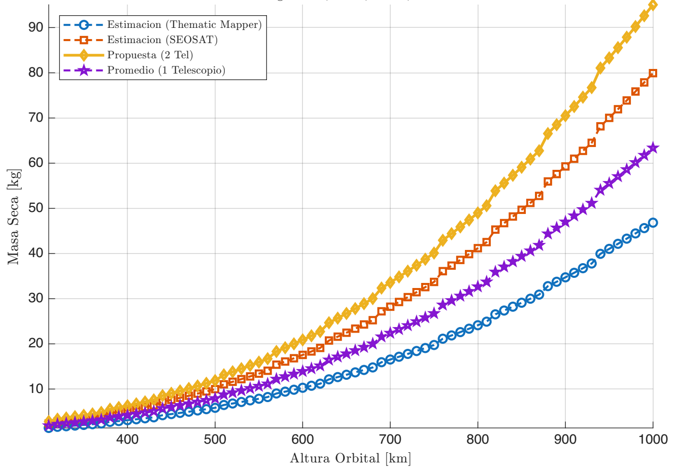
Comparativa de Masa Seca vs. Altura Config: 1 Sat, 2 Tel, Det 1, Korsch
